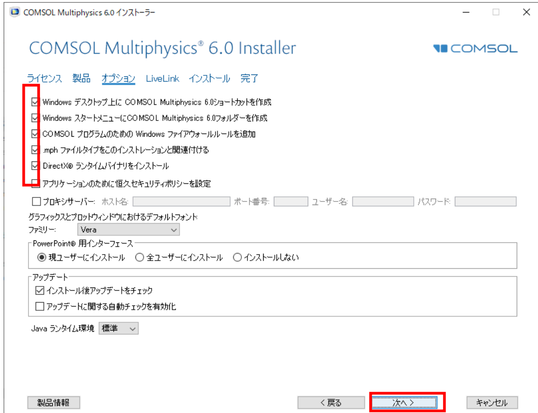
図1.1-5 “オプション”画面
