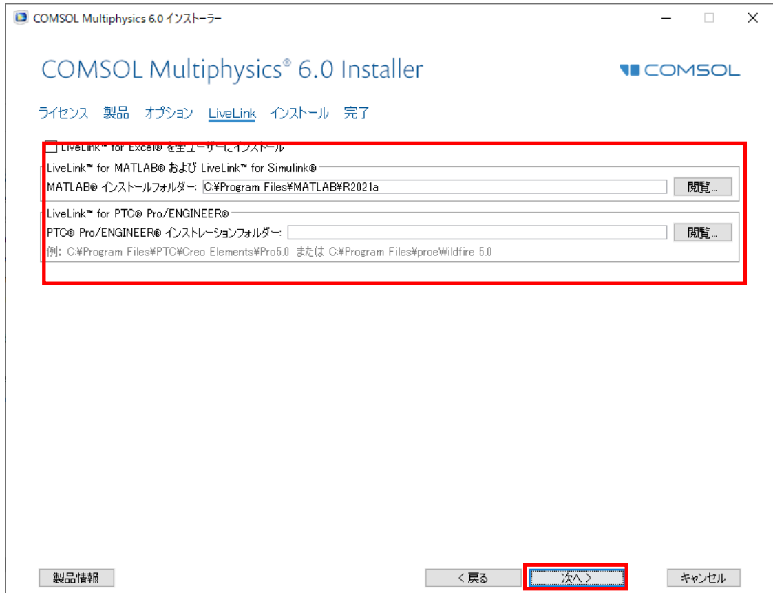
図1.1-6 “LiveLink”画面
