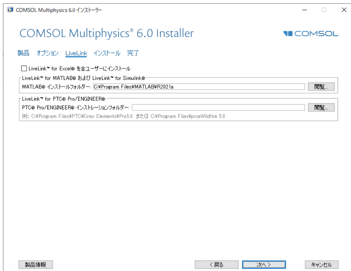
図4.3-5 “LiveLink”画面
