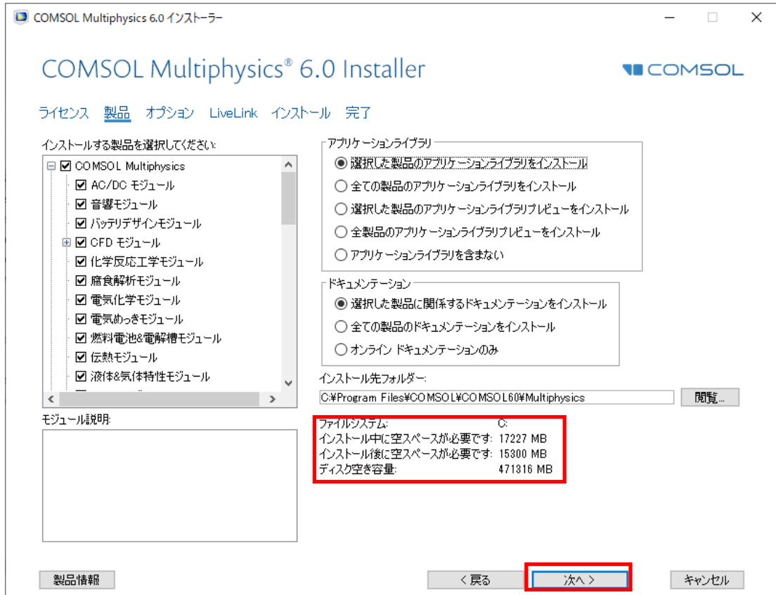
図1.1-4 “製品”画面
