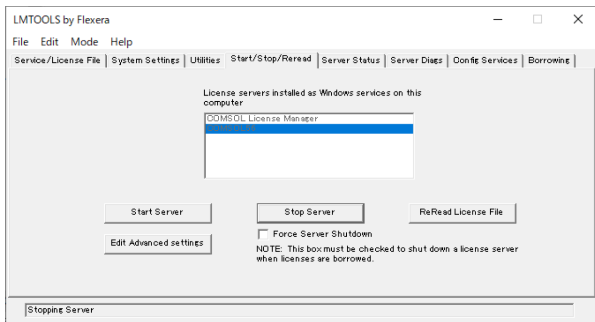
図2.3-7 “Start/Stop/Reread” 画面
