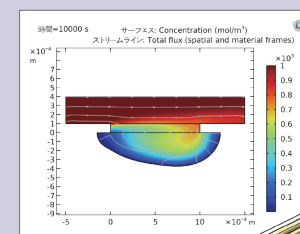
ケミカルエッチング 過程の予測 (層流 + 希釈種輸送)
