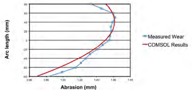
図4. シミュレーション予測と計測によるライニング摩耗との比較
