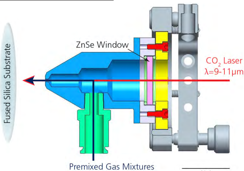
図 3. レーザーベースの CVD プロセスに使用された光学結合のガスノズルを示す回路図。ガスフローが外部ポートを介して挿入してくると同時に IR レーザ光線は ZnSe ウィンドウを介して軸方向に挿入されます。
