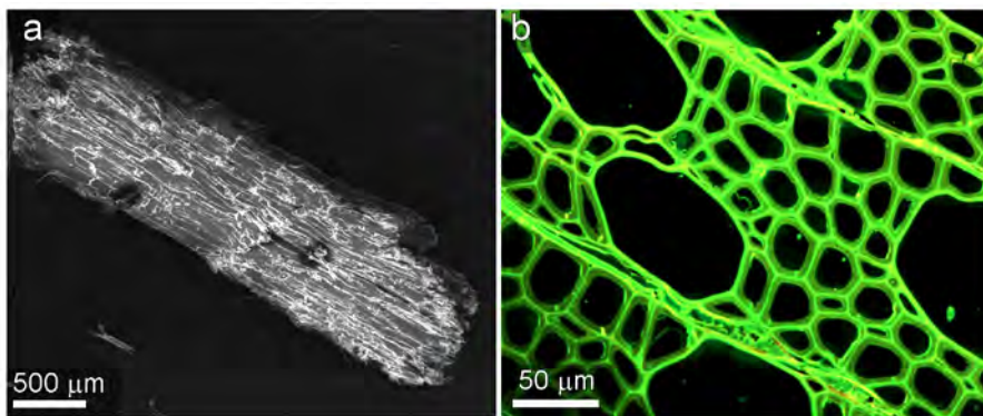
図 2. 左：硬材のバイオマス粒子の形状と構造を明示する走査型電子顕微鏡写真、右：微細構造を示す粒子の横断面の共焦点レーザ走査顕微鏡写真
