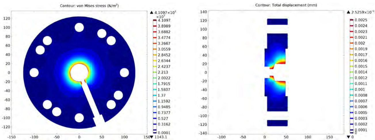
図 7. 型と粘度計保護枠のシミュレーション結果。左：ミーゼス応力曲線 右：全体的な変位のスライス図
