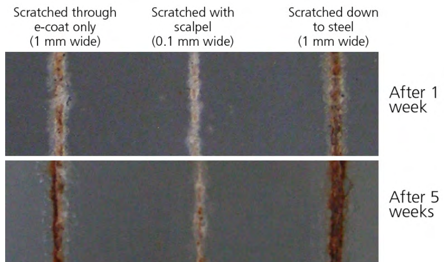
図 4. 損傷した層の中の可視可能な金属腐食を示す亜鉛メッキの施されたスチール製シート上の金属腐食実験 (上から見たもの)。Bösch 氏は、層間剥離プロセスで傷の大きさの影響を分析するために、さまざまな深さと幅の損傷をいくつか作りだした。(上段) 1 週間後の結果および (下段) 5 週間後の結果が示されている。
