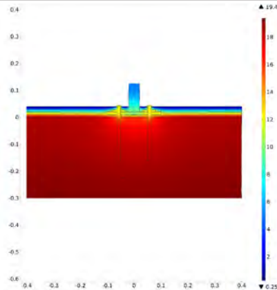
図 4. ブラケットを通した断面の等温分布および温度分布を示すシミュレーション結果
