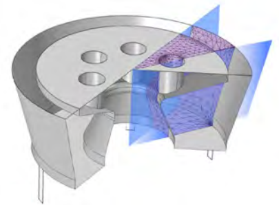
図 2. 4134 コンデンサマイクロフォンのジオメトリ図。セクタ数を削減したジオメトリで用いたメッシュの図であり、ジオメトリ全体の 12 分の 1 が示されている。
