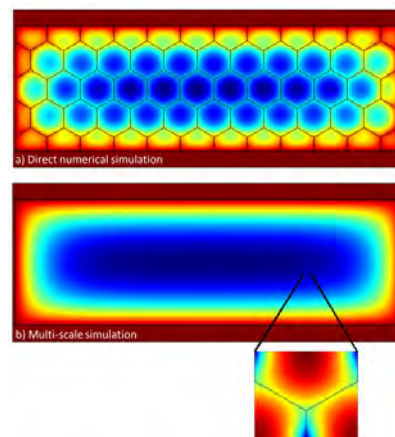
図 3. OLED の光出力を示す COMSOL ソフトウェアのシミュレーション結果。上：六角グリッドを含むモデル 下：均質化された材料特性を持つマクロモデル。
