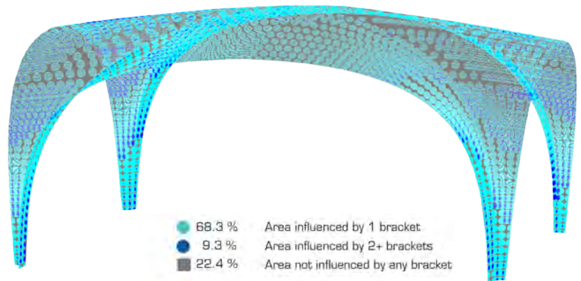
図 5. 1 つのブラケットによる影響、2 つ以上のブラケットによる影響、どんなブラケットにも影響されない、それぞれをハイライトしたエリア 図 2 に表示されたシェル骨組みのモデルの 1 つ
