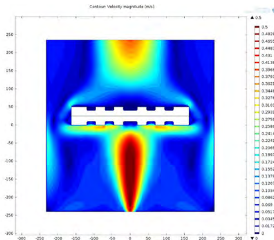
図 4. ベキングプレート周囲の空気の流れ
