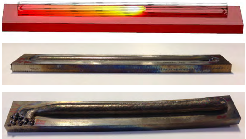
図2. SMDプロセスの間、熱サイクルによって製造部分上に残留応力が引き起こされます。上:SMDパートのシミュレーション 中:1回だけの沈着。目立った偏位は見当たらない。下:6回の沈着。容易にその偏位が分かる。
