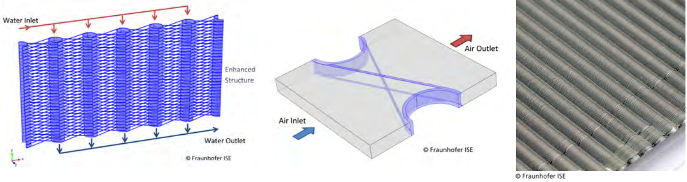
図 3. 左：チューブに注水される温水を示す装置のジオメトリ。冷気は、チューブを通過し、水がチューブを流れる時この水を冷却する。中央：冷気が入り、暖気が出ることを示すシミュレーションジオメトリ。ワイヤー構造およびチューブは紫色で表示されている。右：実験的試験で用いられた装置のジオメトリ
