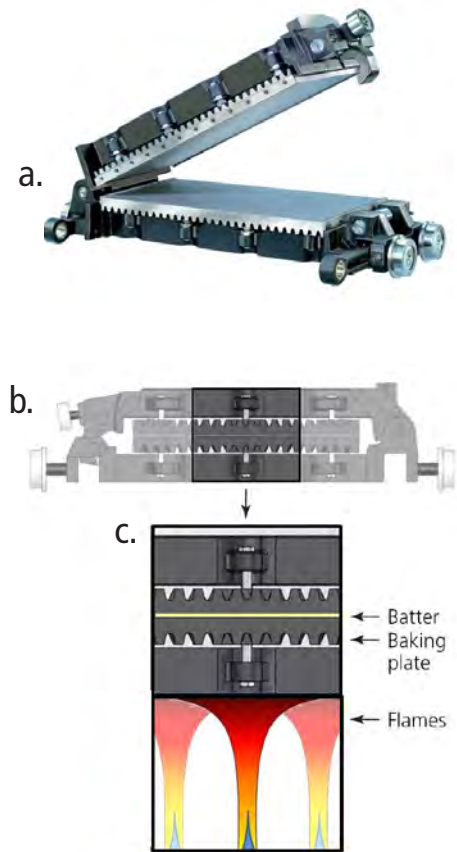
図 3. 2つのウェハー・ベキング・プレート (a) Kit Kat® のウェハーを焼き上げるために使用。(b) 上下のプレートが間の生地を挟み圧搾します。(c) プレートの下の炎は、ウェハーを焼き上げます。
