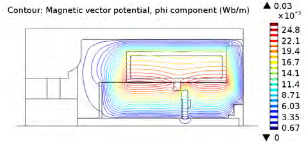
図2. ソレノイドコンポーネントにおける磁気ポテンシャル
