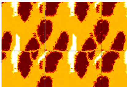
図 2. 求められる異方性熱伝導率のための最適な材料（3種類の材料）構成を示す Barink 氏のシミュレーション結果。このシミュレーションは、高伝導の領域（白）、低伝導の領域（オレンジ）、非導電性材料と空隙の領域（赤）を示しています。いくつかのユニット・セルは周期的に配列されます。
