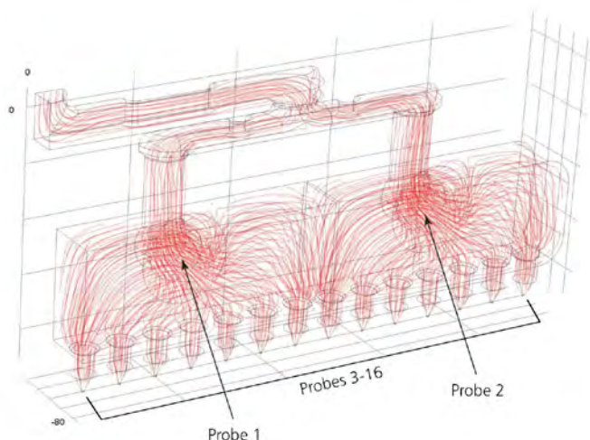
図2. 各ノズルチップと各流路に位置するプローブは、デポジッターとノズルのチョコレート流量と圧力を示し、スペック内で変化しています。流線はチョコレートが流れる方向性を示しています。
