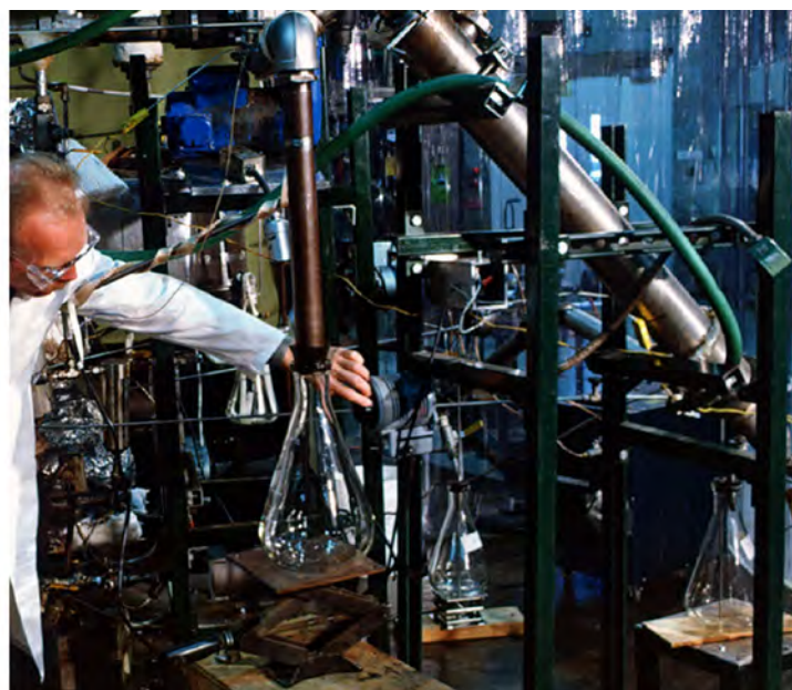
図 1. 熱分解の準備段階において、木質バイオマスは粉碎され（写真左）、さらに化学的処置が施されます。分解の完全なモデルを開発するためには、伝熱、物質伝達、化学反応、相変化などの様々な物理的プロセスを考慮する必要があります（写真右）。この写真は、商用前の化学反応装置における熱分解で生じた圧搾バイオオイルガスを回収するフラスコです。写真提供者：Warren Gretz 氏、NREL 05756（左）、Phil Shepherd 氏、NREL 03677（右）
