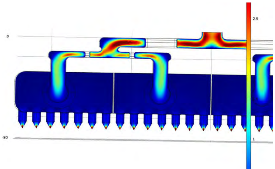
図1. 上：デポジッターの SOLIDWORKS® ソフトウェアジオメトリ 下：COMSOL Multiphysics® シミュレーションデポジッターのノズルと流路内のチョコレートの流れのサイズを示しています。
