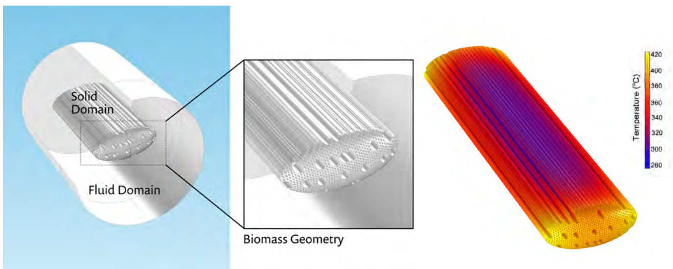
図 3. 左：硬材粒子を囲む流体の特性を表現した COMSOL® ソフトウェアモデルのジオメトリ 右：共役伝熱の過渡シミュレーションが示す温度分布
