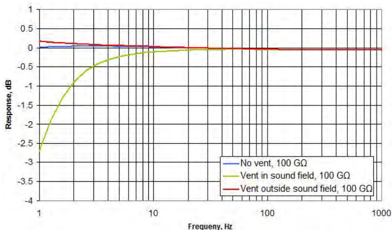
図 5. 空気孔なしの構成の場合、感度が増すのは超低周波ではマイクロフォン内部の音場が完全に等温になるため。音場の外に空気孔がある構成の場合、最初は空気孔なしと同様に推移するが、空気孔が振動板の裏側で圧力を解放し感度がさらに増す。
