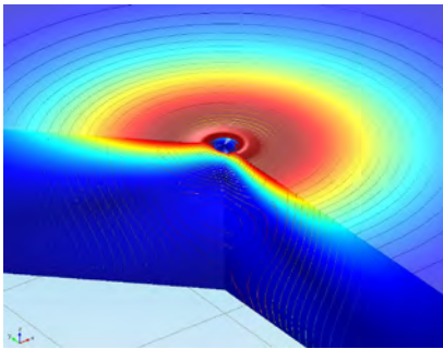
図 2. レーザで加熱されたガラスのマランゴニ流のシミュレーション結果。表面張力レーザー加熱が温度内の勾配を引き起こし、半径方向外側に材料が流れ、さざ波もしくは層のような形を作る場合、この結果が生じます。
