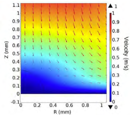
図 4. L-CVD の速度と温度フィールドのシミュレーション。左：速度輪郭は、直径 3mm のノズルからの L-CVD 先駆体フローと空気—ガラスインタフェースのレーザ伝熱により引き起こされた温度フィールドとの関連を示しています。右：蒸発シリカの速度流線型。左下角にガラスの拡散—支配移送を示しています。(濃青)
