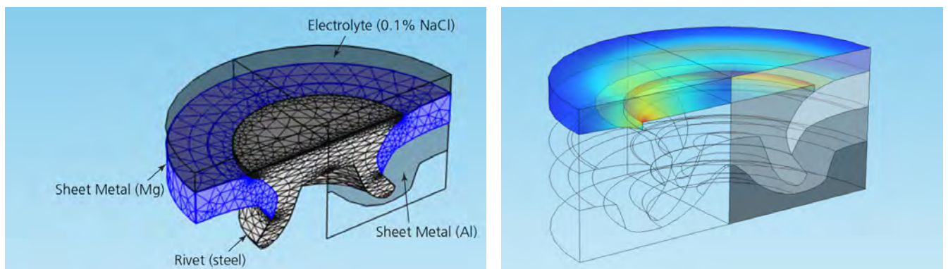
図 2. 左：COMSOL マルチフィジクスソフトウェアで描写されたパンチリベット接合の片側部分のジオメトリ 右：リベットと金属シートの表面における電流密度を示したシミュレーション結果。このシミュレーションは、リベットと金属シートにおける電流を数学的にモデル化したものである。最大の電流密度は鋭角部分（シャープエッジ）で発生している。
