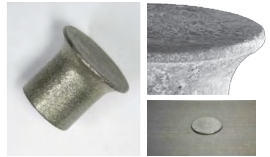
図 1. 左：傷のないリベット 右上：金属腐食のために水酸化マグネシウムの沈着（白色部分の拡大）が生じているリベット 右下：実験用の金属シート内のリベットの拡大図
