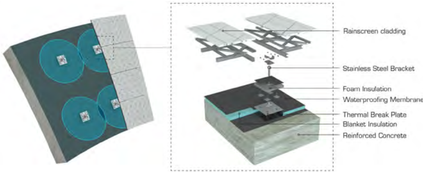
図 3. 固定ブラケットを取り付けたレインスクリーンシステムのハイライトビュー
