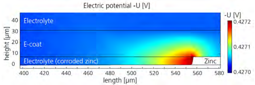
図 5. 左：実験用の金属シートの横断面の拡大図。この金属シートでは、一つの小さな傷が電着および亜鉛層を破損している。右：電着および電解質における電位を示す COMSOL マルチフィジックスソフトウェアの結果。白色の領域は、亜鉛の多くが既に消耗された後に残った亜鉛を示している。
