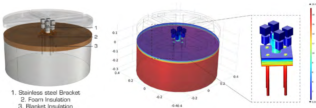
図 6. 左：RhinoCeros® ソフトウェアに組み込まれ COMSOL Multiphysics® にインポートされたブラケットおよび周囲を囲む断熱材の 3次元モデル
