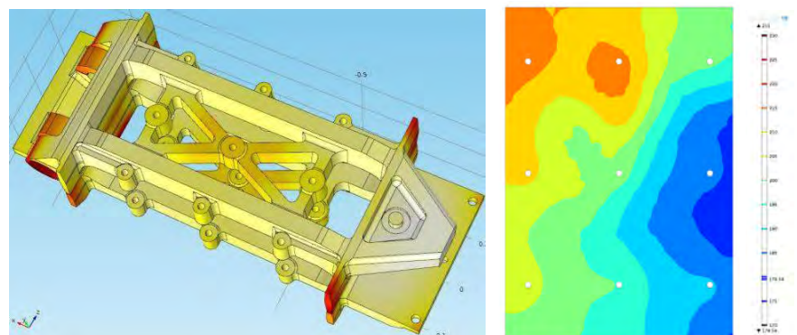
図 5. 左：ベキングプレートの支持フレーム内の温度分布 右：ベキングプレートの表面上部の温度プロファイル。ここではボルトの周囲でより温度が高く、複数箇所にて見られる (白丸部分)
