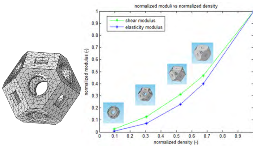
図 4. 左：金属 3D プリンティングの最適化されたセルのメッシュ化モデル 右：様々なセルの設計に対応した均質化材料特性の外観
