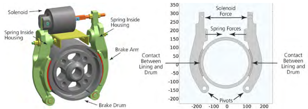
図1. 左：ブレーキのCADジオメトリ、右：ブレーキドラム、アーム、およびピボット、反発するスプリング、ソレノイド力、およびブレーキライニングとドラム間の接触を示しているブレーキライニング摩耗モデルセットアップ
