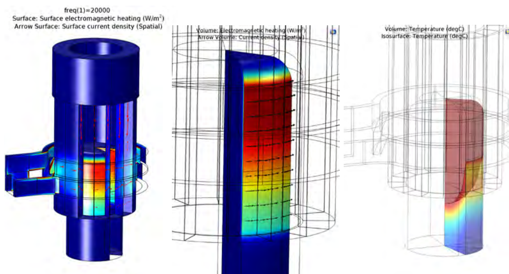
図 2. 冷却るつぼのモデルで、るつぼの電磁加熱 (左)、溶解シリコン (中央) とトリプル-ポイント固体/液体/気体インタフェース (右) の予測に使用されています。赤/黄色は溶解を示し、青/緑は固体の状態を意味しています。
