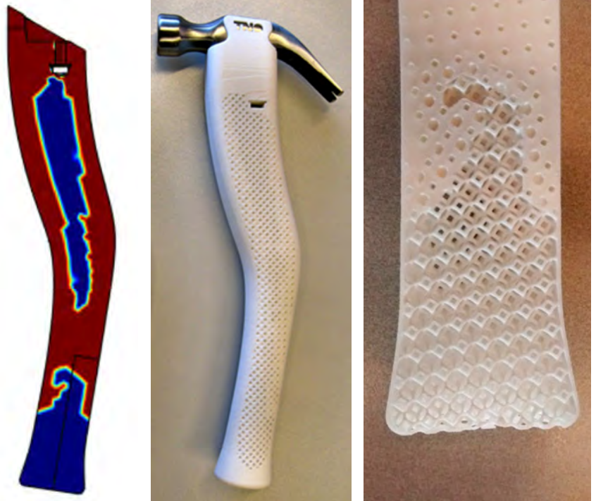
図 5. 左：COMSOL ソフトウェアでのトポロジー最適化の結果 中央：ナイロンでプリントされた最適化ハンマーの柄 右：3 種類の異なるセル型を含むパターンをクローズアップ：上部の近くで小さな穴を持つ高密度セルと下部方向に低密度セルがあり、その間に僅かながら中間体がある。
