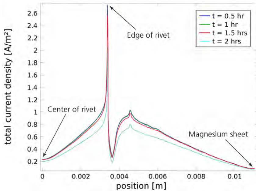
図 3. リベット結合の表面の様々な位置における局所的な電流密度を示す COMSOL ソフトウェアのプロット図
