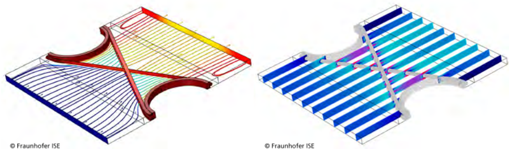
図 4. 左：空気中、チューブ壁、2つのチューブを結合するワイヤーにおける速度流線型および温度分布を示すシミュレーション（赤：暖い；青：冷たい）。右：空気中の速度の大きさを示すシミュレーション
