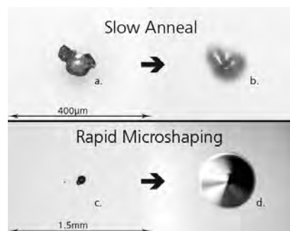
図 1. ハイピーク出力のレーザーパルスに連続的に接触することで生じる光学ダメージの例。光学表面のダメージを (a) と (c) に示します。またそれに伴って生じた修復サイトは (b) と (d) です。ゆっくりとした中間アニーリングは (a) の部分を修復する際に使用され、最近になって NIF で採用開始した素早いミクロ形状技術は (c) の箇所の修復に使用されました。これにより光学的に安全なものになります。
