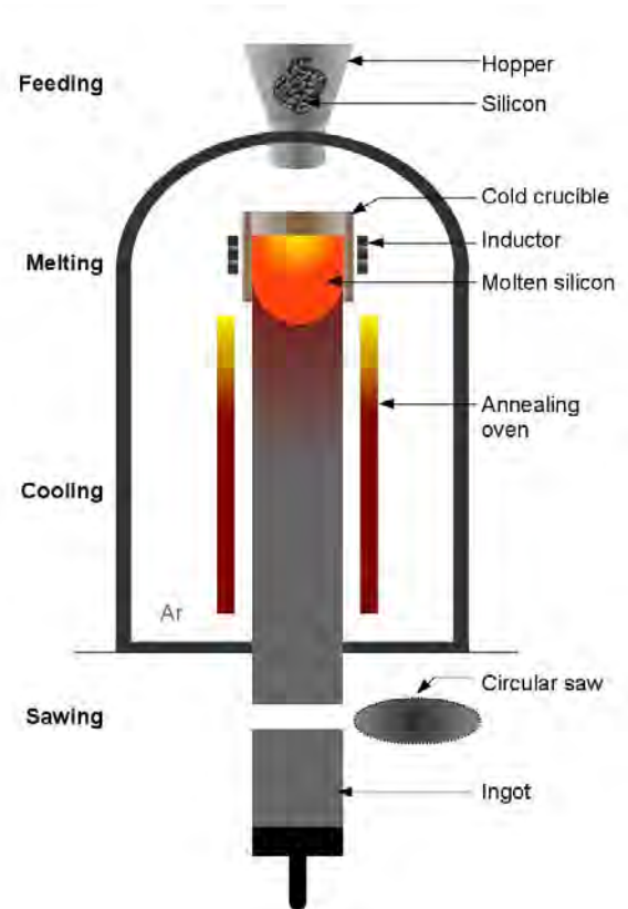
図 1. 回路図は、太陽光発電アプリケーションのシリコン製造時に使用する、継続的に casting し続ける冷却するつぼ (4C) プロセスを示しています。材料のシリコンは、上部にあるホッパーに注がれ、加熱、冷却され、その後インゴットにカットされます。フランス、EMIX
