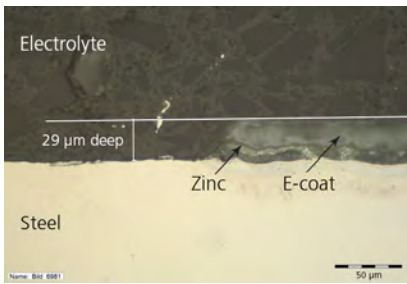
図 5. 左：実験用の金属シートの横断面の拡大図。この金属シートでは、一つの小さな傷が電着および亜鉛層を破損している。右：電着および電解質における電位を示す COMSOL マルチフィジックスソフトウェアの結果。白色の領域は、亜鉛の多くが既に消耗された後に残った亜鉛を示している。
