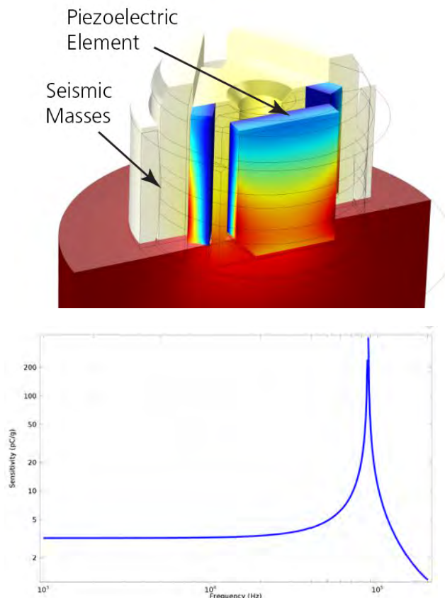
図 6. 吊下げ型圧電振動トランスデューサのシミュレーション結果。上：圧電部品と振動物質における機械的変位および電場。下：トランスデューサの最初の共振が約 90 kHz で生じることを示す周波数応答のグラフ。この機器での計測は、90 kHz よりもかなり低い周波数のものだけを対象とすべきである。
